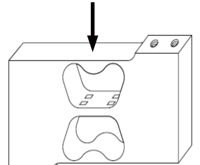
■SPI [型過負荷保護機能付]
